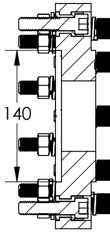
SECTION A-A SCALE 1 : 4
